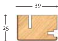
Art. 3013 Montante telaio Frame stile
