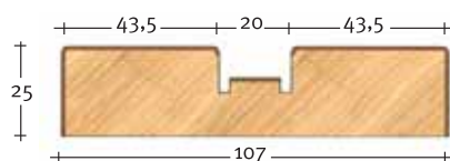
Art. 3008 Montante battuta Rabbet stile
