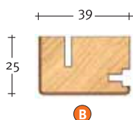
Art. 3013 Montante telaio Frame stile
