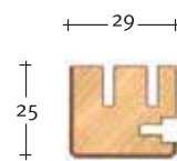
Art. 3012 Montante telaio Frame stile
