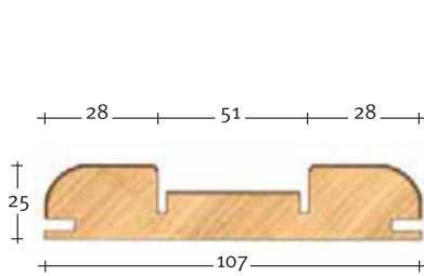
Art. 3045 Montante battuta Rabet stile
