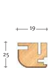
Art. 3062 Montante telaio Frame stile
