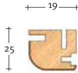
Art. 3062 Montante telaio Frame stile
