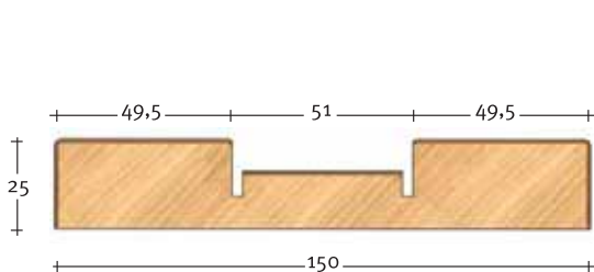
Art. 3005 Montante battuta Rabbet stile
