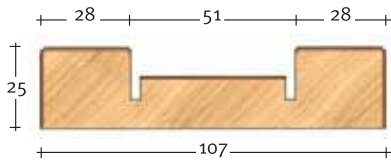
Art. 3001 Montante battuta Rabbet stile
