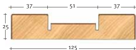
Art. 3004 Montante battuta Rabbet stile
