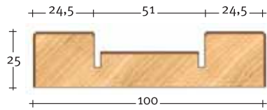
Art. 3003 Montante battuta Rabbet stile
