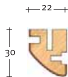
Art. 3017 Montante telaio Frame stile
