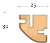
Art. 3060 Montante telaio Frame stile
