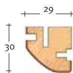
Art. 3060 Montante telaio Frame stile
