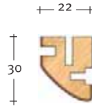
Art. 3017 Montante telaio Frame stile
